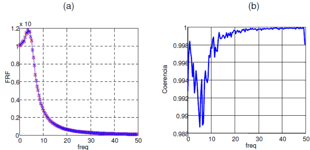
Figura 6.5. (a) Comparação de H(f) teórico ('—') com estimadores \hat{H}_1 ('o-') e \hat{H}_2 ('x-') para n = 4096 , nb=16 ; N=256 usando um amortecimento 5 vezes maior. (b) Função coerência.
